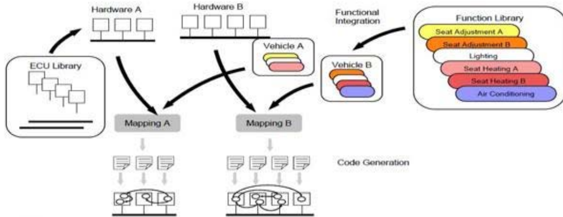
شکل ۳: اهداف AUTOSAR
